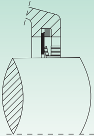
Obturator de anillo en v "TSNA" para: SNG-SNU "TSNA" v-ring seal for: SNG-SNU
