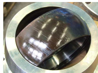
Ložiskový celok ZLK LC 110/190 2RS po skúškach
