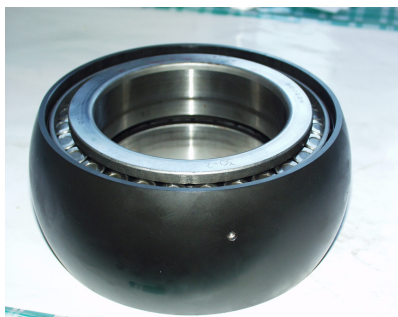
Ložiskový celok ZLK LC 110/190 2RS po skúškach
